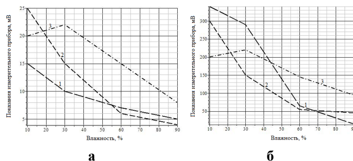
Рис.8. Зависимость влияния весовой влажности на КСВ измерительной антенны: (а) от влажности почвы с саранчой; (б) от влажности почвы без саранчи.
