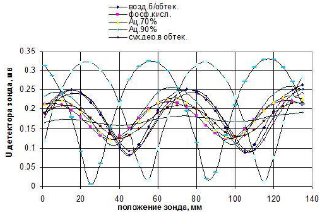
Рис.3. Калибровочные измерения КСВ дипольной антенны.
