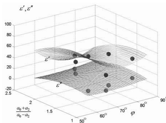
Рис.4. Модель зависимости \varepsilon' = f_1\left(\frac{a_0 + a_2}{a_0 - a_2}\right), \varphi и \varepsilon'' = f_2\left(\frac{a_0 + a_2}{a_0 - a_2}\right), \varphi .
