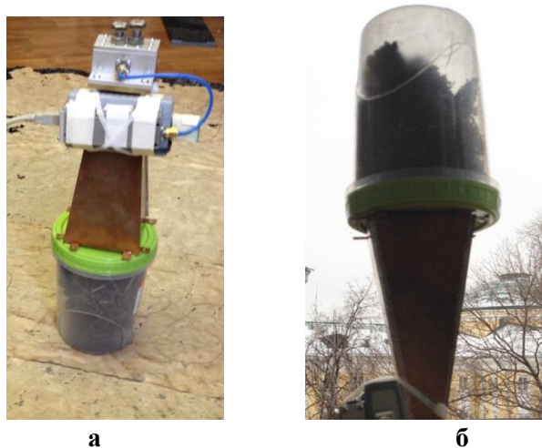
Рис.6 Использование радиометра 4см диапазона для обнаружения кубышек в лабораторных условиях: а) на фоне черного тела; б) на фоне атмосферы.
