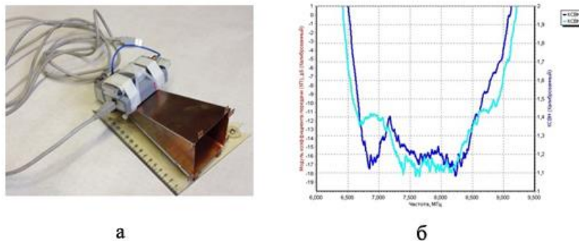
Рис.5. Радиометрические исследования: а – внешний вид радиометра; б – частотная характеристика для двух режимов.
