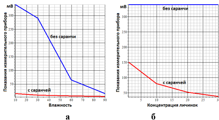
Рис.7. Зависимость влияния весовой влажности и концентрации личинок на КСВ измерительной антенны: (а) от влажности почвы при концентрации личинок 10% ; (б) от концентрации личинок при влажности 60% .
