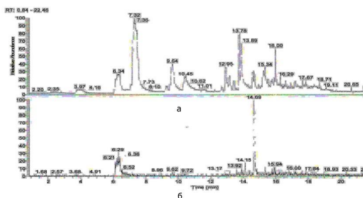
Рис.9. Масс-хроматограммы личинок а) по полному току, б) по характерному току m/z 93.
