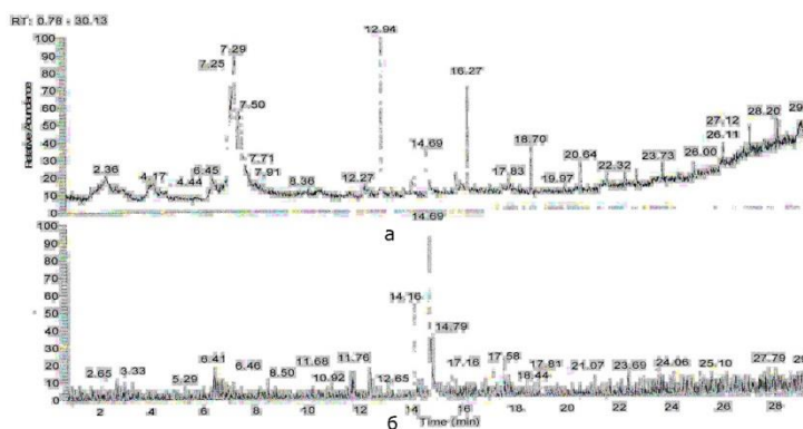
Рис.10. Масс-хроматограммы почвы а) по полному току, б) по характерному току m/z 93.
