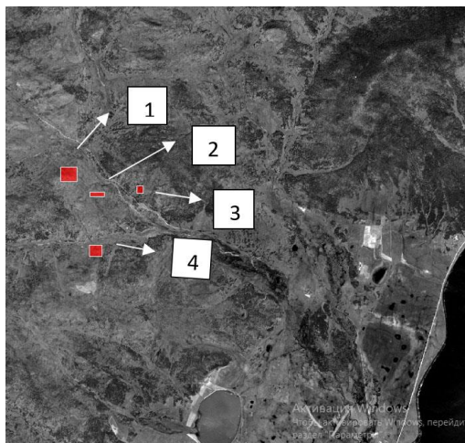
Рис. 2. Расположение тестовых площадок, объединенных в 4 группы
