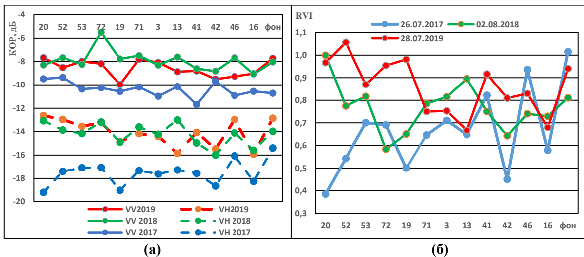
Рис. 3. Изменение коэффициента обратного рассеяния (а) и RVI (б) для тестовых участков за 2017-2019 годы
