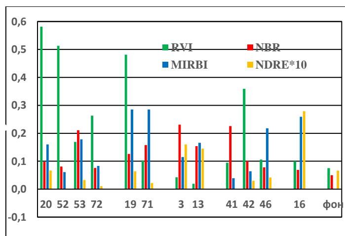
Рис.7.Изменение значений по абсолютной величине радарного и спектральных индексов для исследуемых площадок
