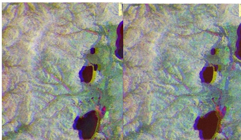
Рис. 4. Изображения исследуемой территории в RGB кодировке: red-26.7.2017, green – 2.8.2018, blue – 28.7.2019
