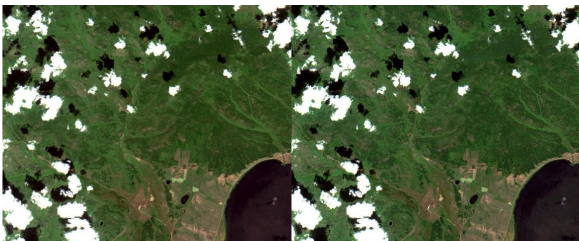
Рис. 9. Сравнение двух изображений S2 в естественных цветах (каналы B2, B3, B4) дата съемки 26.7.2019 до (а) и после(б) атмосферной коррекции
