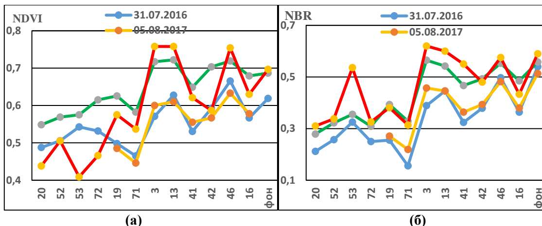
Рис. 5. Изменение NDVI (а) и NBR (б) для тестовых площадок за 2016-2019 годы
