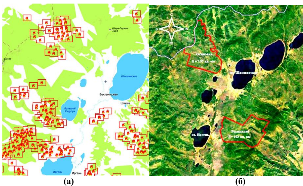
Рис.1. Карта пожаров за 14.4.2015 (а), расположение модельных площадей для исследования динамики изменения растительных сообществ (б)
