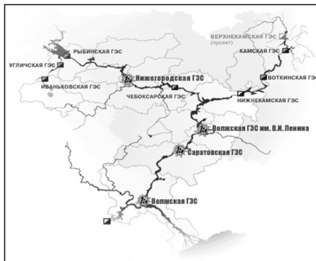
Рис.1. Волжско-Камский каскад водохранилищ
