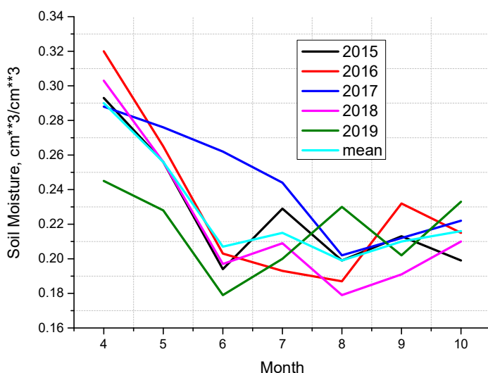
Рис.3. Сезонный ход среднего значения влажности почв Волжского бассейна в 2015-2019 годах
