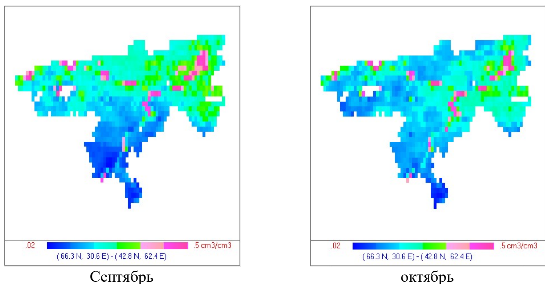
Рис.2. Влажность почв Волжского бассейна по данным SMAP измерений в 2015 году
