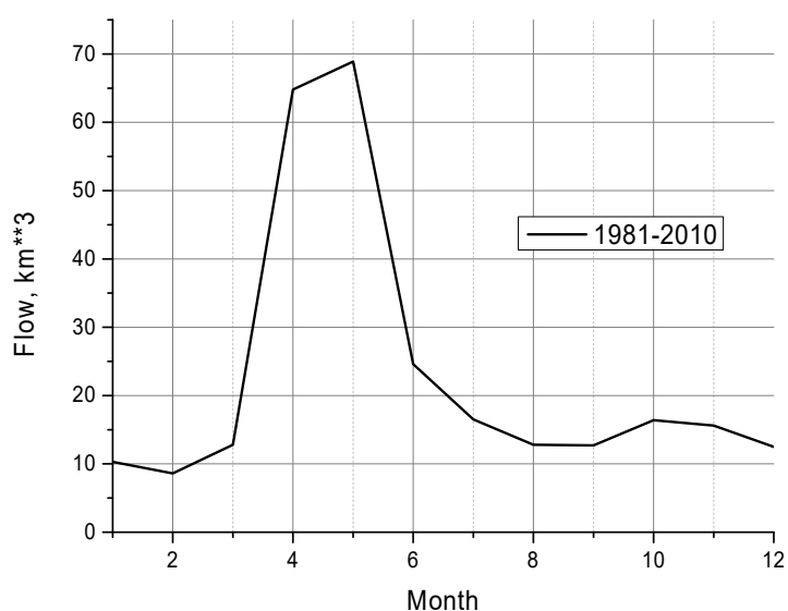
Рис. 4. Многолетний сезонный ход стока Волги
