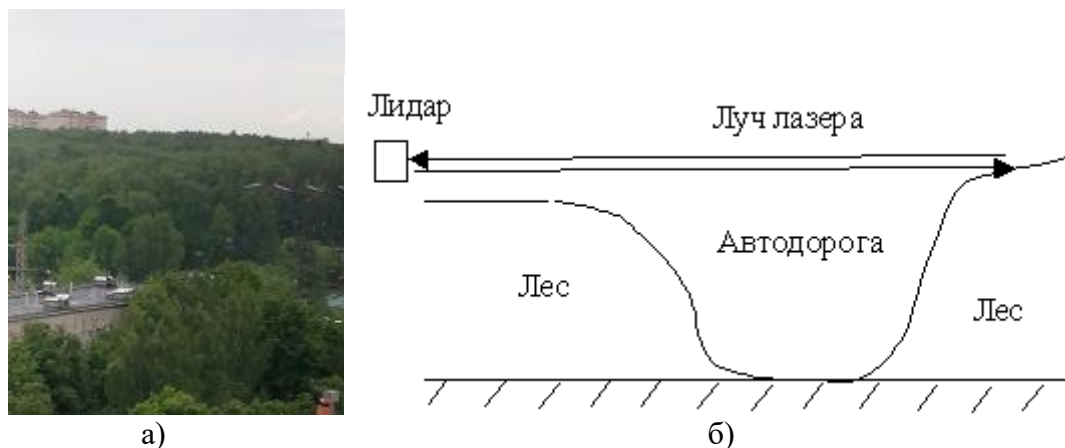
Рис.3. а) фотография трассы 2.25 км, б) профиль подстилающего ландшафта
