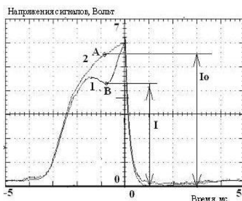
Рис.2. Пример осциллограммы сигналов после фотоприемника. Кривая 1 – сигнал при отражении светового излучения от объекта (деревьев), расположенных на расстоянии 2.25 км, 2 – сигнал при отражении светового излучения от близкорасположенной (~0.5 м) мишени
