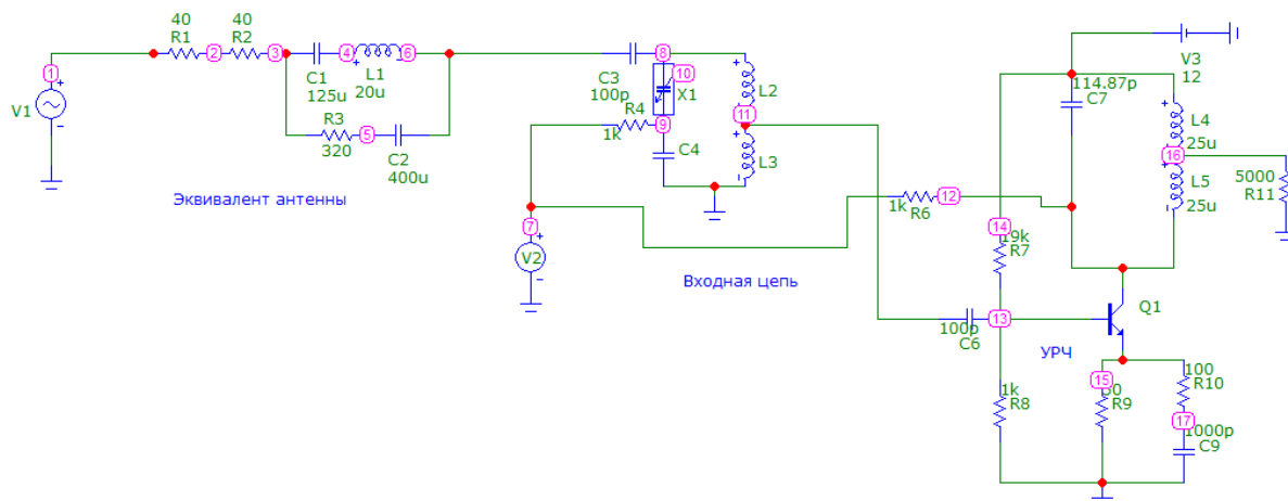
Рис. 1 – Принципиальная схема схмотехнической модели экспериментального стенда
